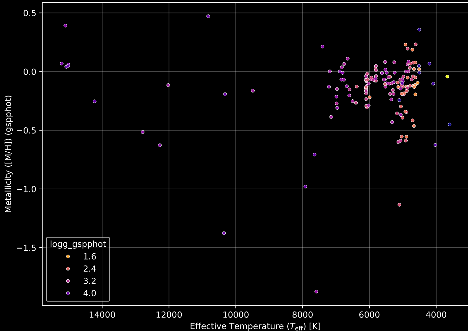
APOGEE DR17 Field: [184-04] Stellar Population Parameters (n= 157)
